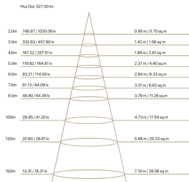
Gráficos y curvas de distribución lumínica
